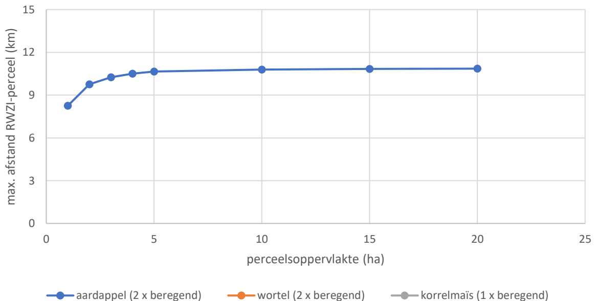
Figuur 27. – Maximale transportafstand RWZI – perceel, indien enkel in juli beregend wordt met over de weg aangevoerd effluent. Bij elke beregeningsbeurt wordt 25 L/m 2 beregend, ofwel 250 m 3 /ha. Indien een perceel van 5 ha aardappelen 2x beregend wordt, bedraagt de maximale afstand perceel – RWZI 10,7 km, opdat beregenen rendabel is. De lijnen voor wortel en korrelmaïs staan niet op de figuur omdat transport voor deze teelten in deze situatie nooit rendabel is.
