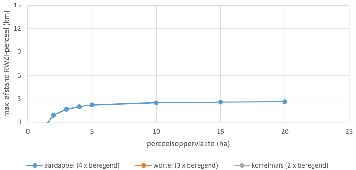
Figuur 26. – Maximale transportafstand RWZI - perceel, indien het volledige voorjaar beregend wordt met over de weg aangevoerd effluent. Bij elke beregeningsbeurt wordt 25 L/m 2 beregend, ofwel 250 m 3 /ha. Indien een perceel van 5 ha aardappelen 4 x beregend wordt, bedraagt de maximale afstand perceel - RWZI 2,5 km, opdat beregenen nog rendabel is. De lijnen voor wortel en korrelmaïs staan niet op de figuur omdat transport voor deze teelten in deze situatie nooit rendabel is.
